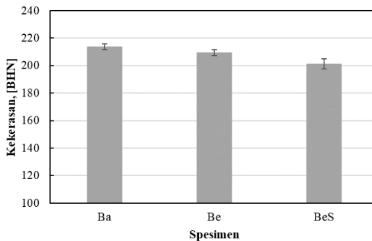
Gambar 4. Kekerasan pada ketiga spesimen.
