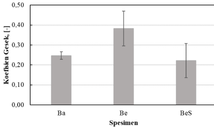
Gambar 7. Koefisien Gesek Steady State pada ketiga spesimen.
