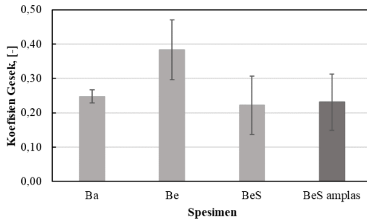
Gambar 11. Koefisien gesek spesimen sebelum dan sesudah perlakuan pengamplasan.
