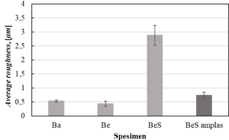
Gambar 10. Kekasaran permukaan spesimen sebelum dan sesudah perlakuan pengamplasan.
