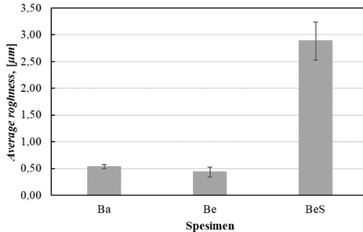
Gambar 5. Kekasaran permukaan pada ketiga spesimen.
