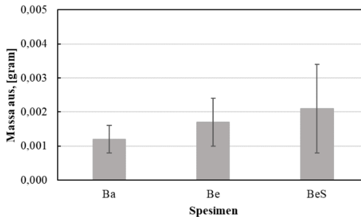
Gambar 8. Massa aus pada ketiga spesimen.
