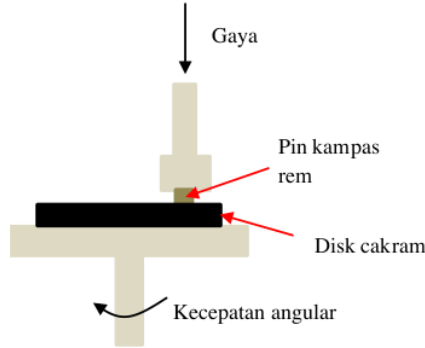
Gambar 3. Skematik uji tribometer pin-on-disk.
