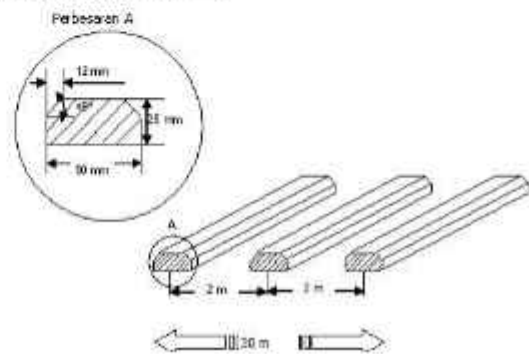
Gambar 2. Balok Pengujian.
