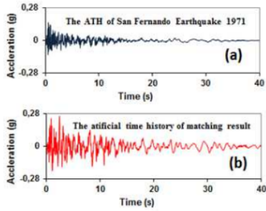
Figure 13. Time history actual (a) dan artifisial (b).
